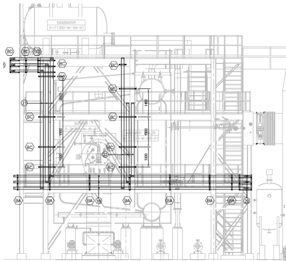
설비 계통 상세도 (계속)
